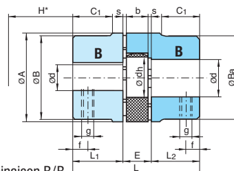
Combinaison B/B
