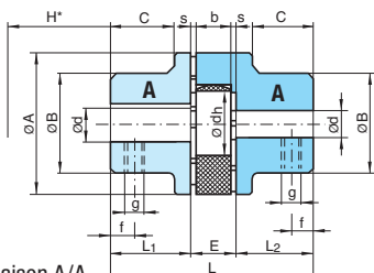
Combinaison A/A
