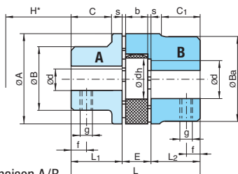
Combinaison A/B
