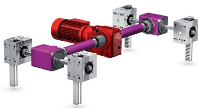
Levage 4 points avec renvois d'angles
