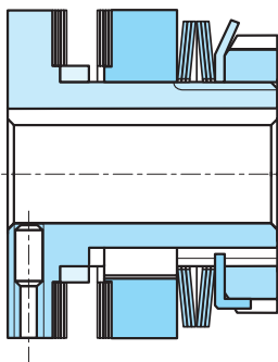
Série mini LC 382 de 2,2 à 9 Nm
