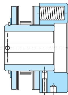
Série haut de gamme à couple constant LC 393 de 2 à 1000 Nm
