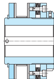
Série standard LC 390 FORME B de 1600 à 12000 Nm
