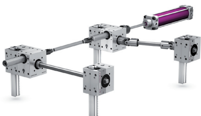
Levage avec cardan ESLR/LRC
