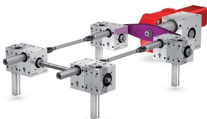
Levage 4 points + ESLR 53
