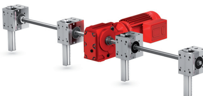
Levage par motoréducteur
