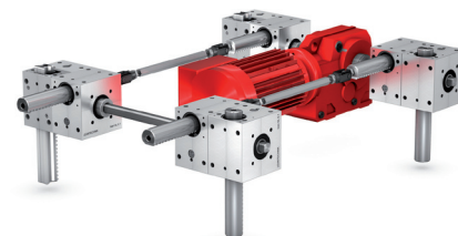
Levage 4 points par motoréducteur
