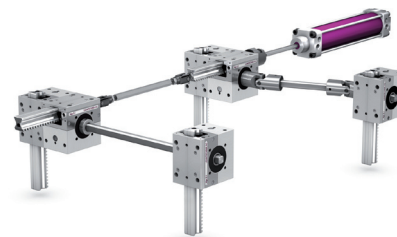
Levage avec cardan
