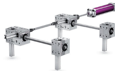
Système de levage LRC
