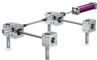
Système de levage ESLR
