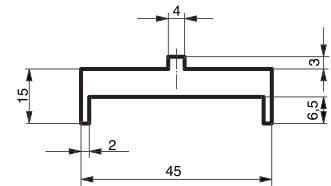
Profil 45x18 Extrudé
