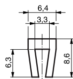
Profil U 6,4x8,6 Extrudé
