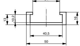
Section O40x8 Usiné
