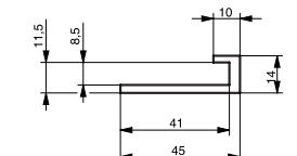
Section O40x8 Usiné
