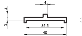
Profil 40x7,5 Extrudé
