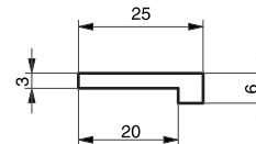
Profil L GE25x6 Usiné
