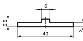
Profil en talon 40x5,5 Extrudé
