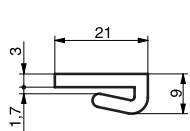
Profil 21x9 Extrudé
