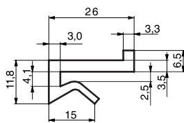
Profil L 26x11,3 Extrudé
