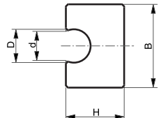
Profil RK (Ø8 ; Ø10 ; Ø12)
