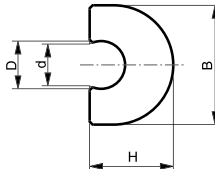
Profil RR (Ø8 ; Ø10 ; Ø12)
