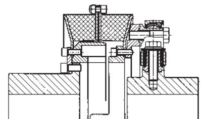
Liaison de 2 arbres avec 2 éléments
