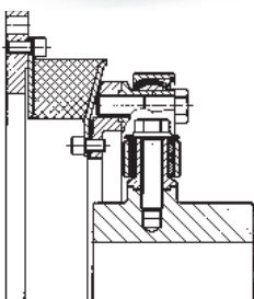
Liaison volant-arbre avec 1 élément
