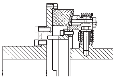
Liaison de 2 arbres avec 1 élément
