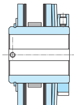
Série standard LC 390 FORME A de 3,5 à 1900 Nm
