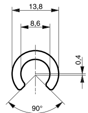
Profil Snap 10
