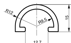
Profil Snap 12,5
