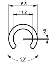
Profil Snap 12,5
