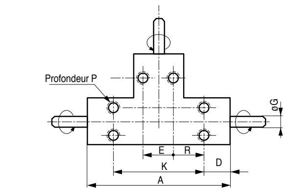
Renvoi en T - RAP.T 6 trous de fixation sur 2 faces RAP.T possibilité de 2 arbres de sortie tournant à l'opposé
