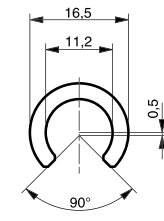
Profil Snap 12,5
