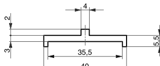
Profil 40x7,5 Extrudé
