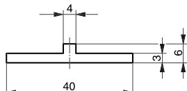
Profil GN 40x6 Extrudé/Usiné
