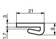
Profil 21 x 9 Extrudé
