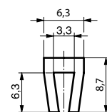
Profil U 6,3 x 8,7 Extrudé
