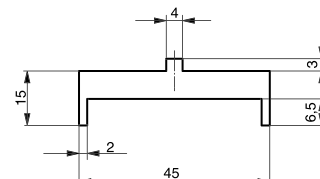
Profil 45x15 Extrudé
