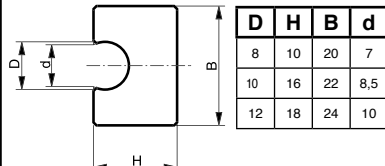
Profil RK (Ø8 ; Ø10 ; Ø12)
