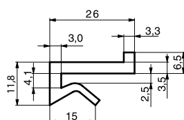
Profil L 26 x 14,8 Extrudé
