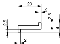
Profil Z GZ20 x 8 Extrudé/Usiné
