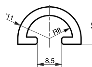
Profil Snap 10
