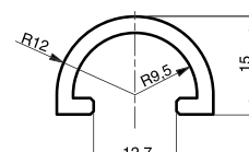
Profil Snap 12,5
