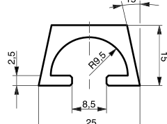
Profil RR (Ø8 ; Ø10 ; Ø12)
